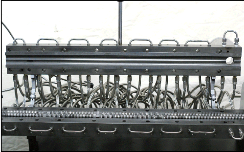
Clam Shell Type Barrel. 바렐을 위로 열면 Screw와 시료를 볼 수 있다.
