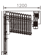
C-20 측면도
