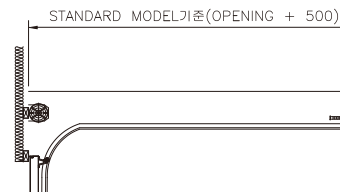
C-30 측면도
