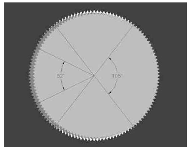
그림 4. Power 시리즈의 치형접촉
