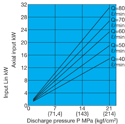
Axial Input
