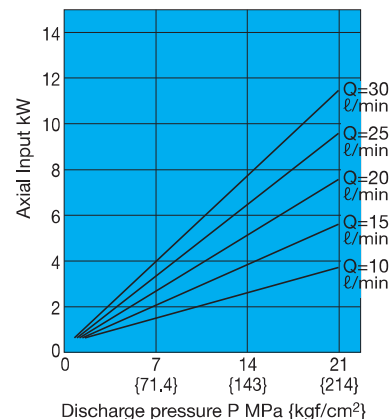
Axial Input
