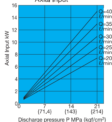
Axial Input
