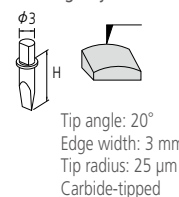
Knife edge stylus
