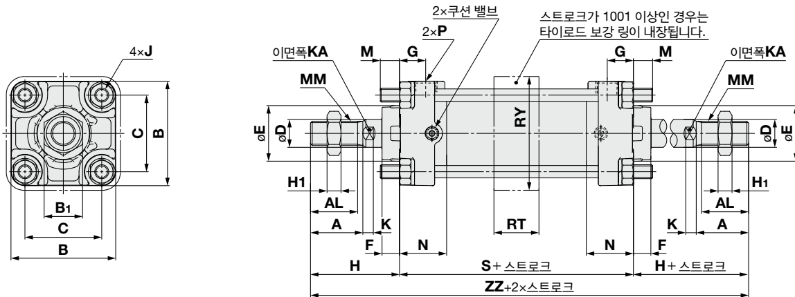
편측 벨로스 부착
