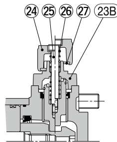
매뉴얼 해제 Lock타입: 추가기호 L
