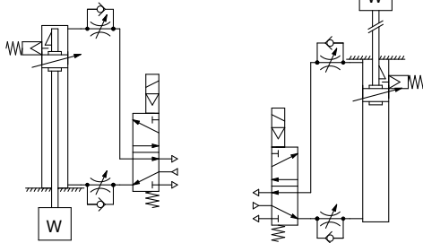
헤드측 Lock 부착
