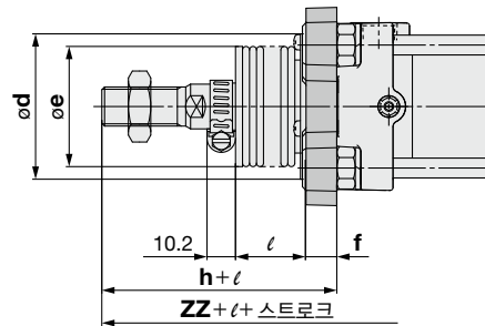
벨로스 부착
