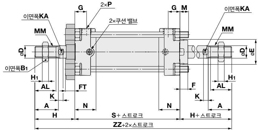
벨로스 부착
