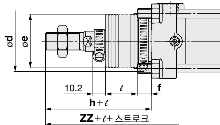
벨로스 부착
