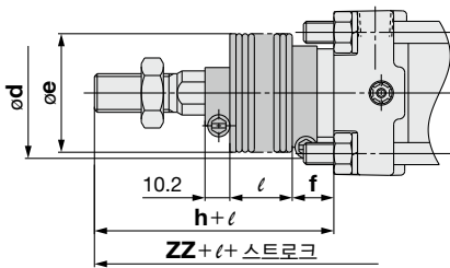
벨로스 부착
