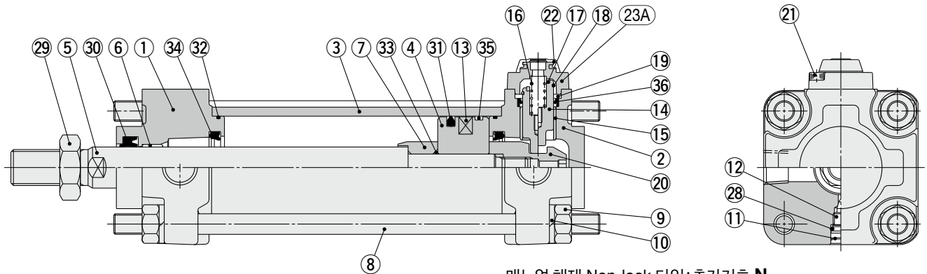
매뉴얼 해제 Non-lock 타입: 추가기호 N
