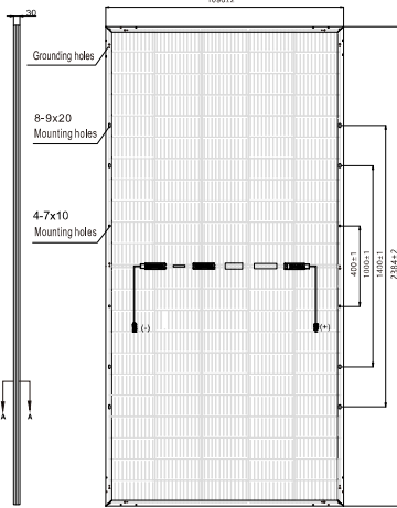
태양광 모듈 치수 Unit: mm
