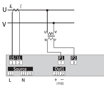
1P2W(LLType)
