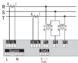
3P3W(LLType)
