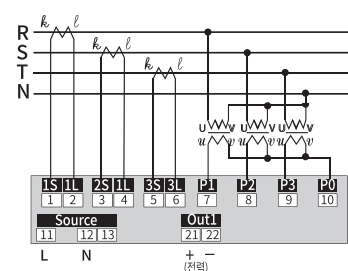
3P4W(LLType)
