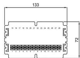
온도계 후면도
